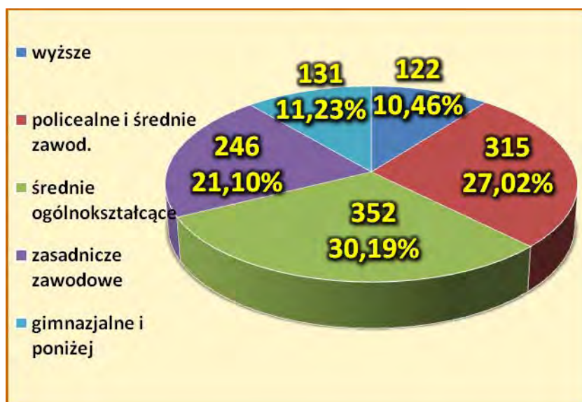
Wykres 3. Osoby bezrobotne do 25 roku życia w podziale na wykształcenie w 2012 r.
